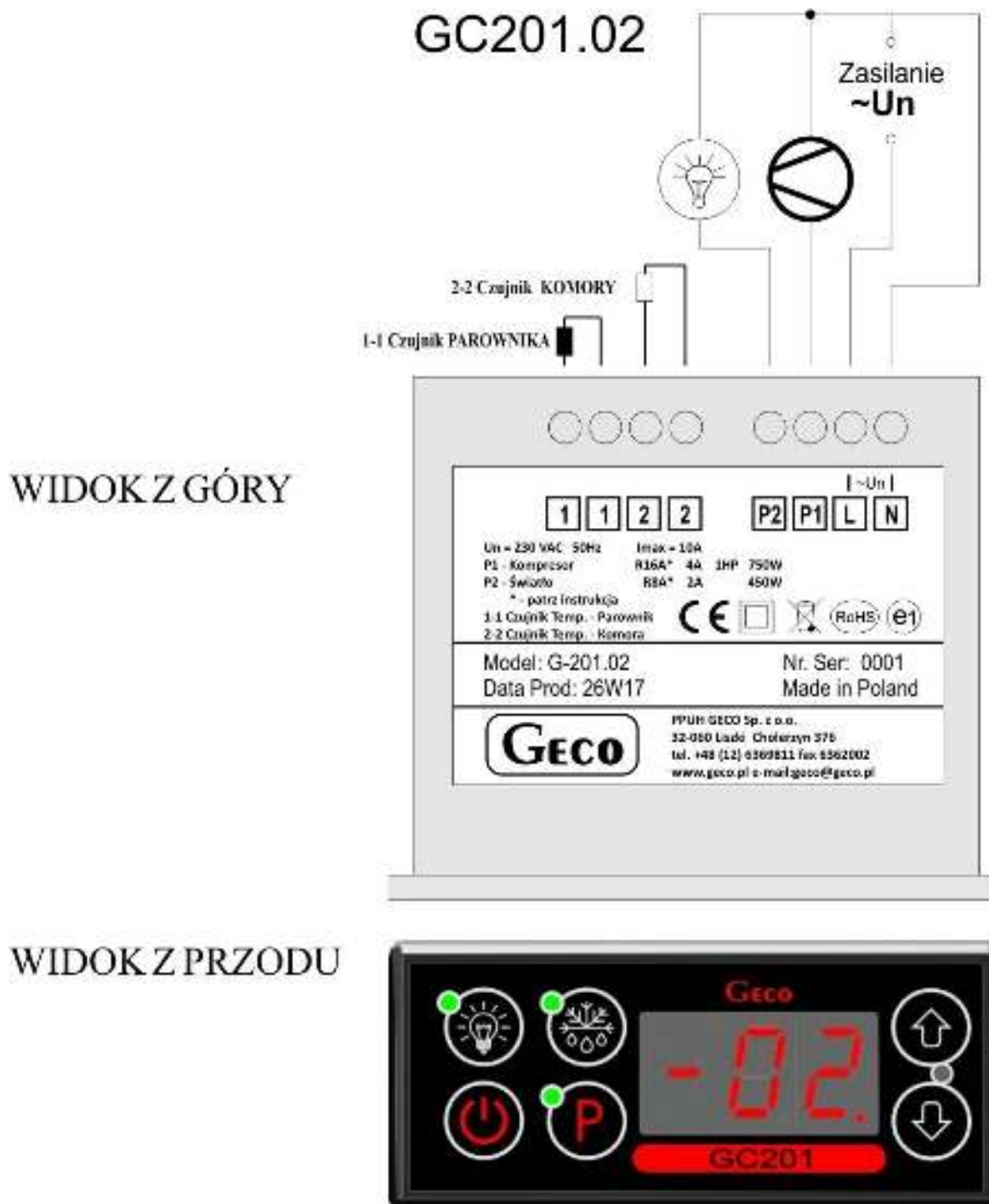
Rys. 4 Schemat podłączenia urządzeń i czujników do modelu regulatora GC201.02, który jest dodatkowo wyposażony w przycisk obsługi oświetlenia.
